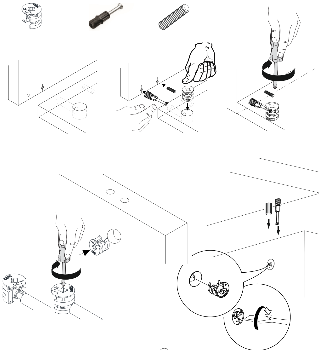
Minifix šroub/skrutka
