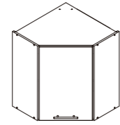
T12/G60NW š × h × v (v mm) 600 × 600 × 720
